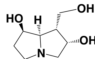
(-)-rosemarinecine
