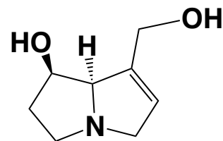
(+)-retronecine
