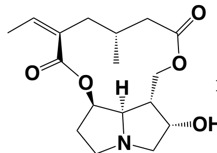
(+)-retronecine
